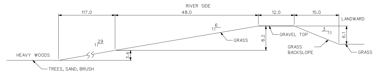
SECTION 3-4 SCALE: 8"=1'-0"
