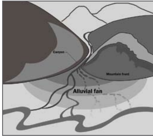
Alluvial Fan
